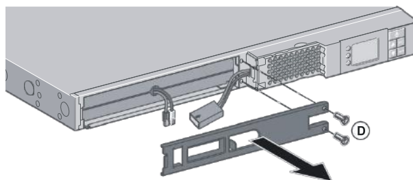
D Снимите металлическую защитную крышку в передней части аккумулятора (открутите два винта)
